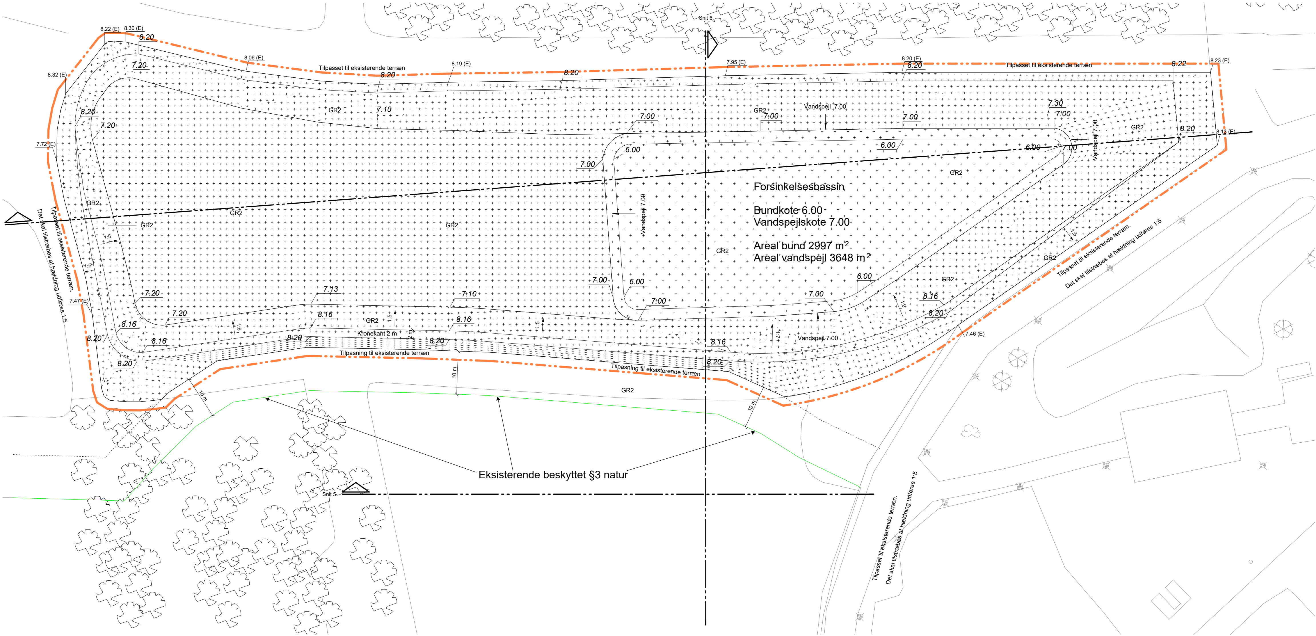
Forsinkelsesbassin og vold - Dependent 1 | 1 : 500
